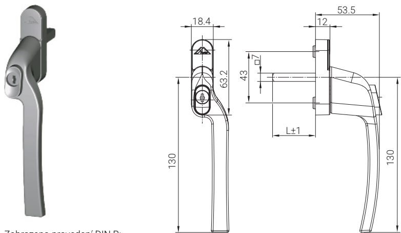
Zobrazeno provedení DIN R; DIN L je zrcadlově obrácená
