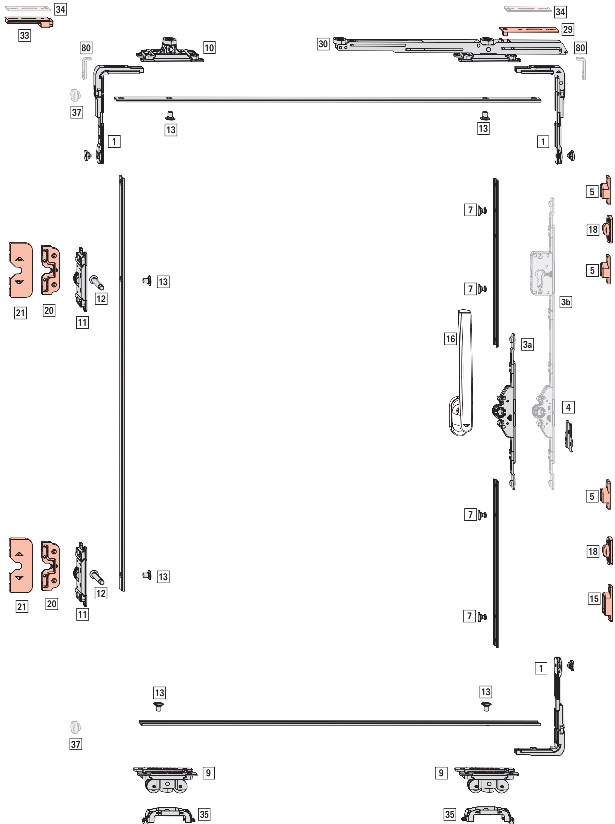
ill.. 4.3: Zházorněno: provedení pravé; FB 900 mm; FH 1900 mm; převod DM 25
