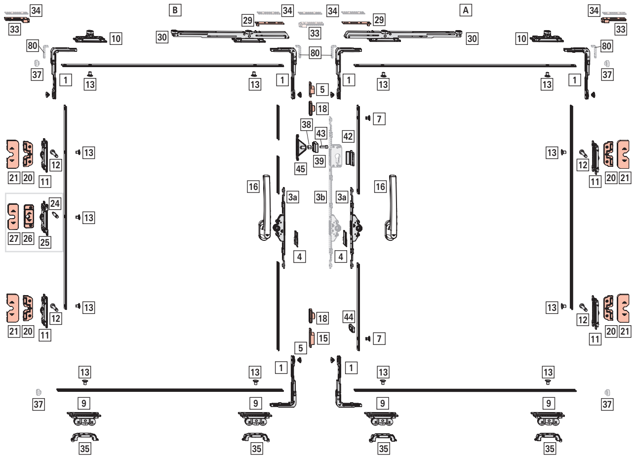
ill. 4.6: Znáznorněno: [A] první v řadě otvírané křídlo provedení L, [B] křídlo otvírající se jako druhé provedení R; FB 900 mm; FH 1300 mm; převod DM 25; řídicí jednotky s funkcí SoftClose
