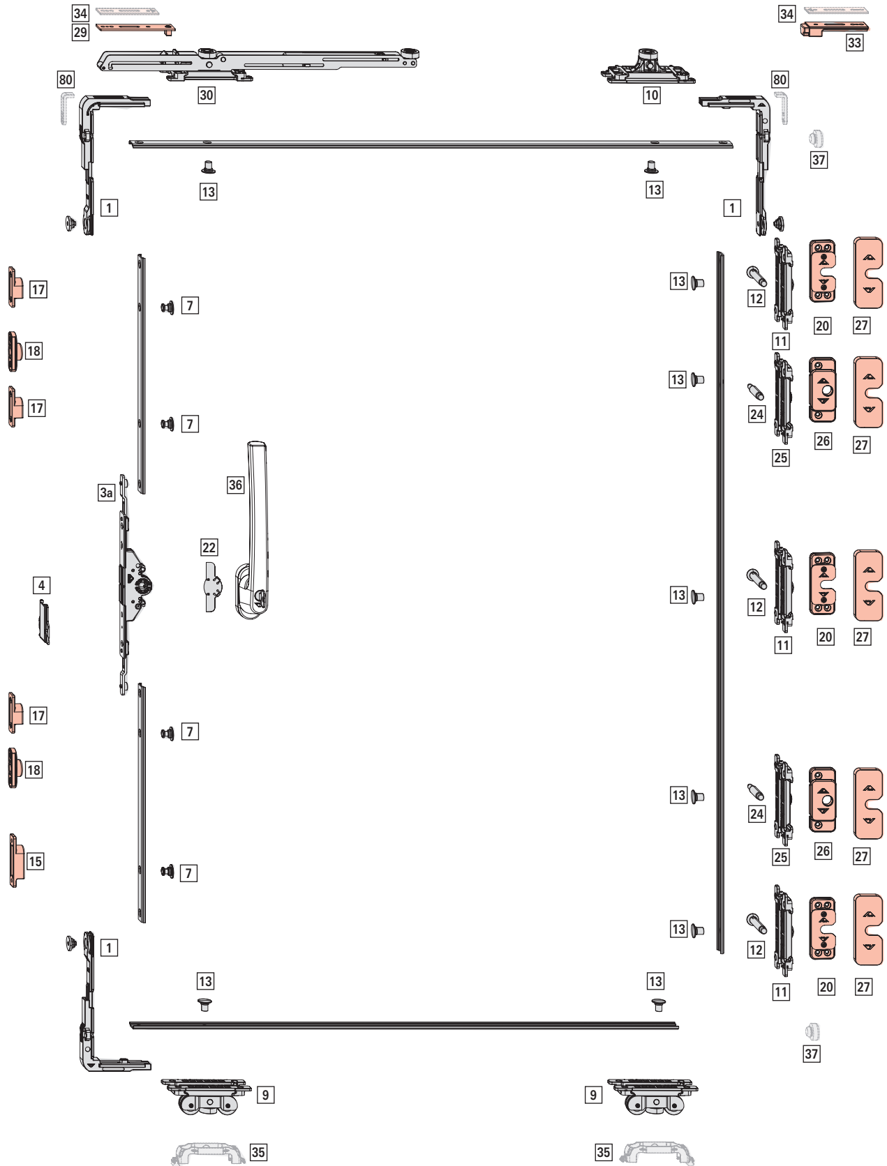
ill.. 4.2: Znážorněno: provedení levé; FB 900 mm; FH 1900 mm; převod DM 25; RC 2
