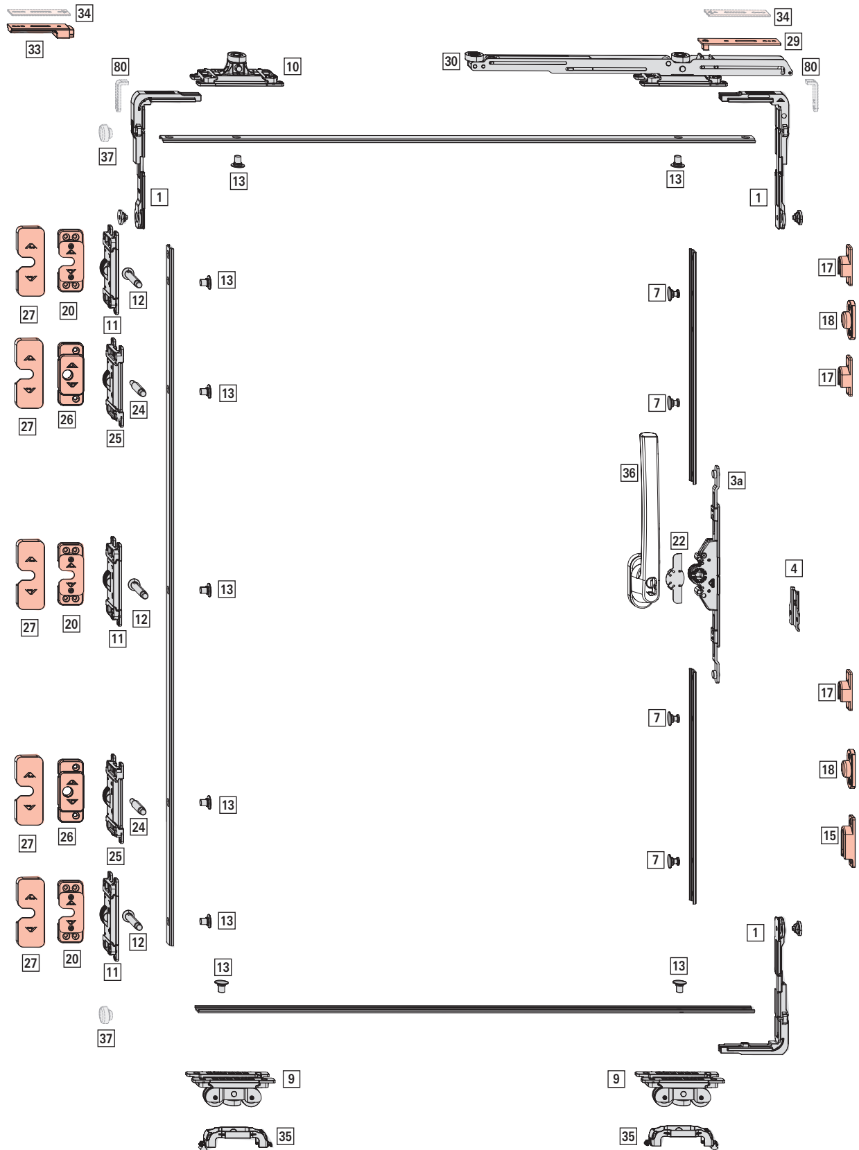
ill.. 4.4: Zházorněno: provedení pravé; FB 900 mm; FH 1900 mm; převod DM 25; RC 2
