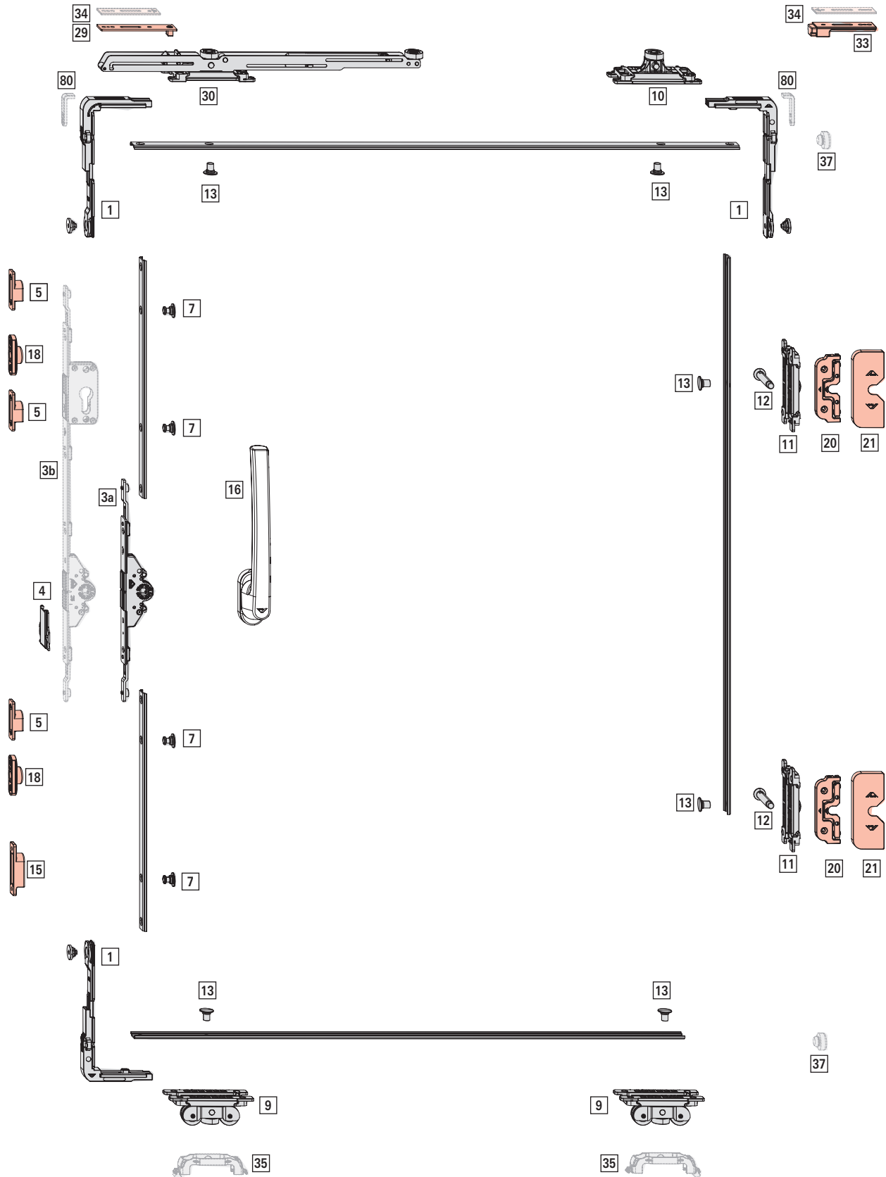
ill.. 4.1: Znáznorněno: provedení levé; FB 900 mm; FH 1900 mm; převod DM 25; FG 150 kg; řídicí jednotka se SoftClose
