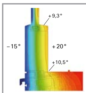
Pevná část U_f hodnota 1,0 W/m 2 K u dřevěných křidel
