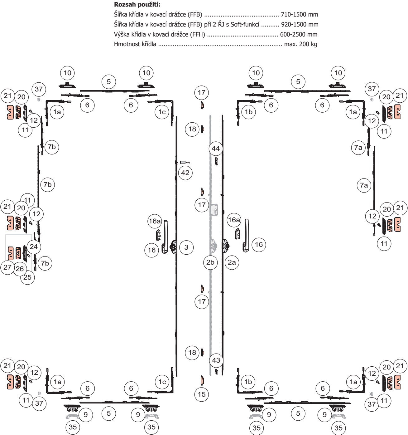
Volitelně (možnosti umístění řídicí jednotky)
