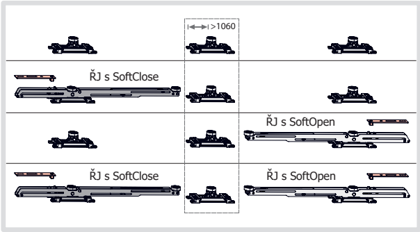
Volitelně (možnosti umístění řídicí jednotky)
