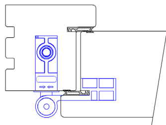
panelové
