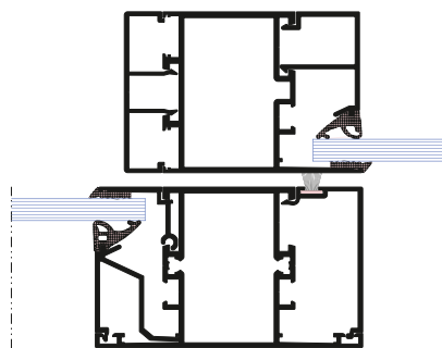
Řez sloupkem
