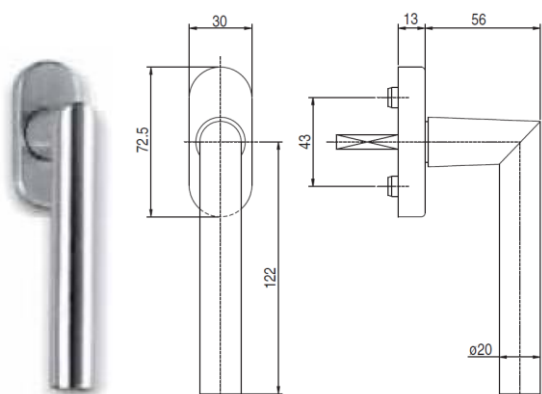
Výkres klik v barvách 9016, 8019, F1, F2, F3, F4, F9
