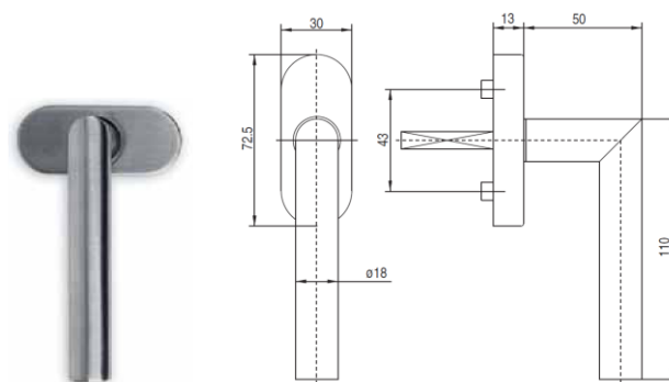
Výkres klik v nerezovém provedení
