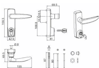
EXTERIÉROVÁ KLIKA S VLOŽKOU
