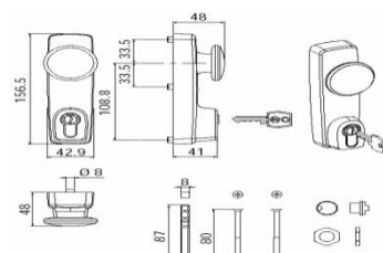
EXTERIÉROVÁ KOULE PEVNÁ S VLOŽKOU
