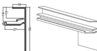
AL koncovka před omítkou PROM (pod omítku)
