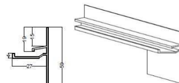
AL koncovka po omítkce POOM (k omíce)
