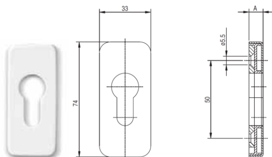
rozeta s překrytím z nerezové oceli
