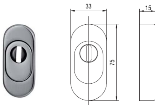
hliníková rozeta s překrytím
