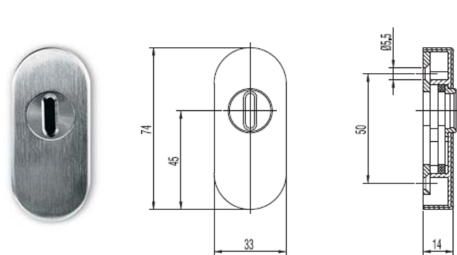
rozeta s překrytím z nerezové oceli
