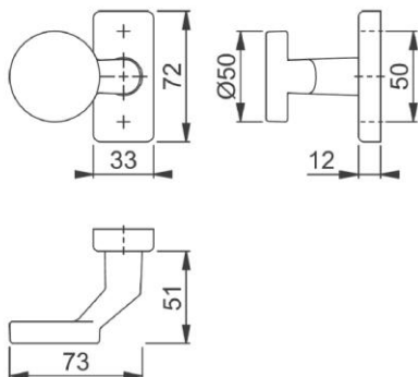
knoflík 58G/55 černá F9714M
