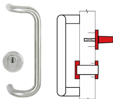
madlo typ G +kulatá rozeta K15P (ilustrativní obrázek)
