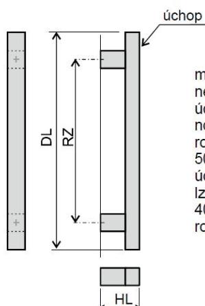
zobrazený model typ FHR30x20-500/350 bez podložek
