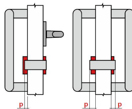
p = výsuv zámkové vložky
