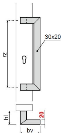
zobrazený model typ KHR30x20-425 včetně hranatých podložek 40x40
