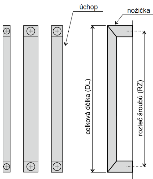
zakončení madla k rámu dveří (detail nožiček)
