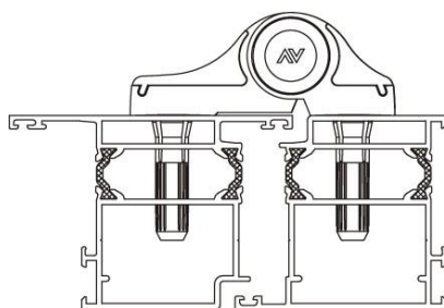
HLINÍKOVÉ HMOŽDINKY
