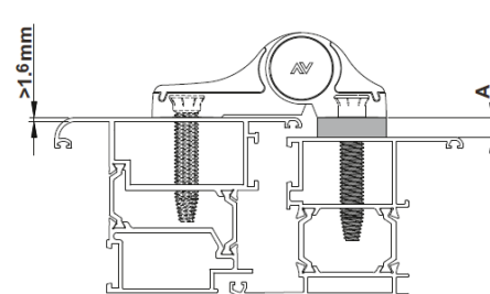
VYROVNÁVACÍ PODLOŽKY
